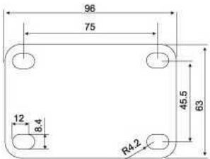
平板 Top plate
