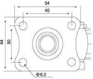
平板 Top plate
